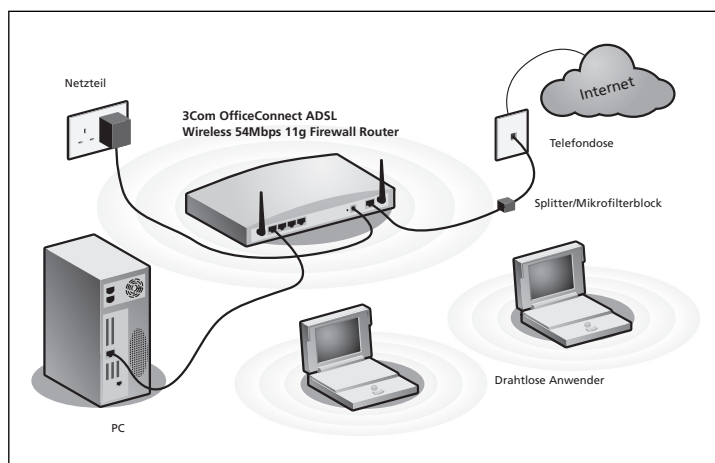
Beispielnetzwerk mit OfficeConnect ADSL Wireless 54 Mbps 11g Firewall Router
