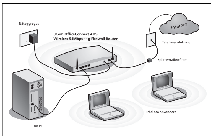
Exempel på nätverk med OfficeConnect ADSL Wireless 54 Mbps 11g Firewall Router
