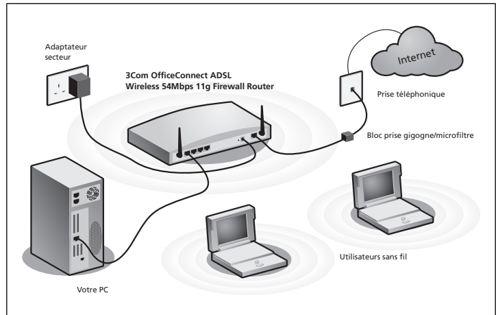
Exemple de réseau avec routeur OfficeConnect ADSL Wireless 54 Mbps 11g Firewall Router
